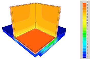
Pont thermique en 3D
