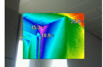
Thermographie
